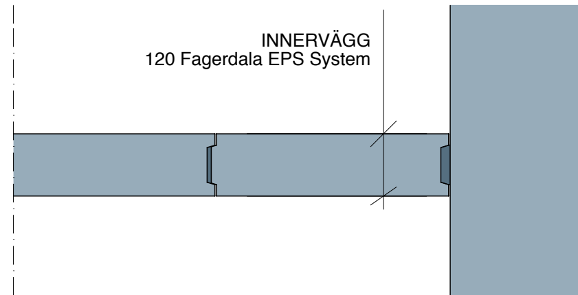
INNERVÄGGSSYSTEM HORISONTALSNITT
