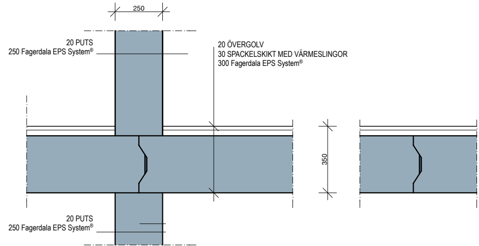
ELEMENTSKARV MELLANBJÄLKLAG
