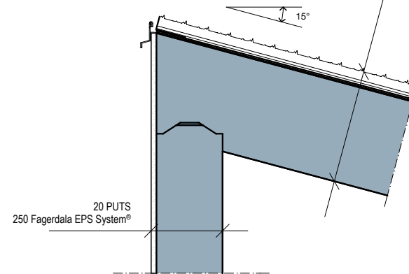
TAKNOCK PULPETTAK
