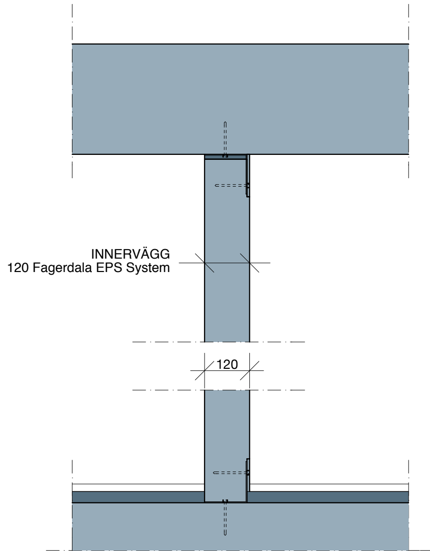
INNERVÄGGSSYSTEM VERTIKALSNITT
