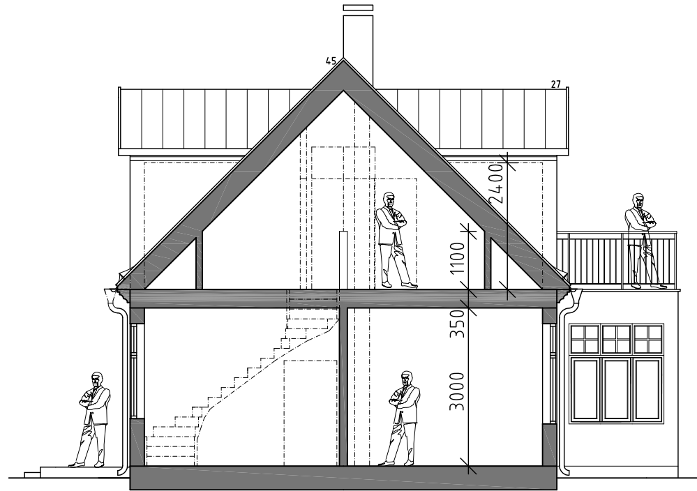
SEKTION
