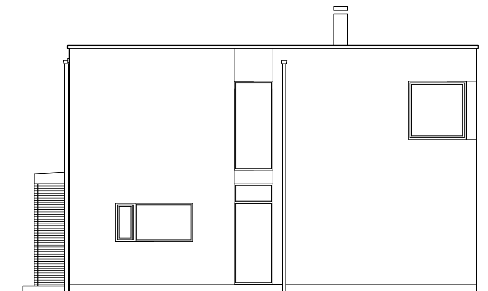
SIDOFASAD 2
