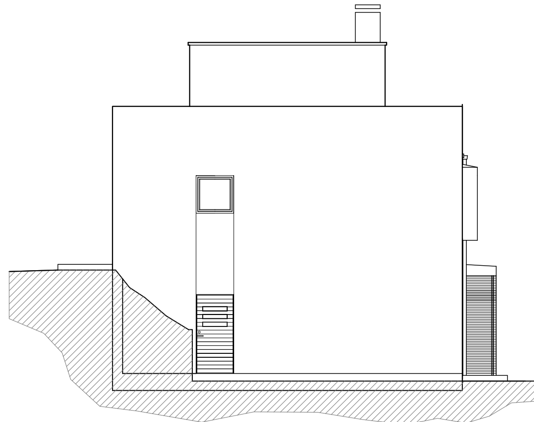
SIDOFASAD 1
