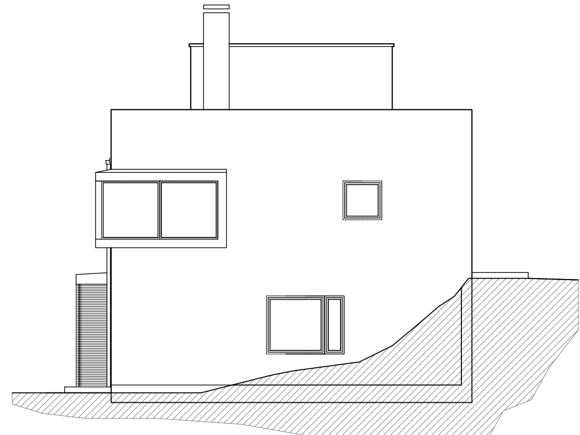
SIDOFASAD 2
